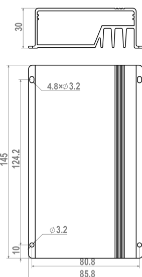
SMR-MPPT1575
