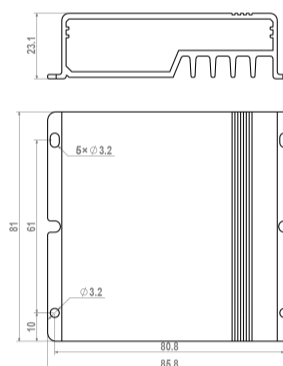
SMR-MPPT1050
