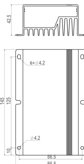
SMR-MPPT2075
