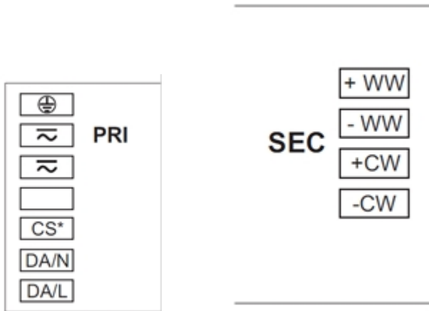
Anschlüsse am LED-Treiber für LLE G2 PRE Module
