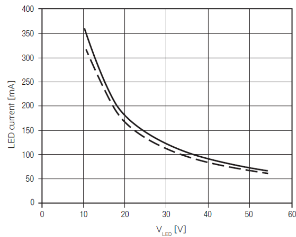
EM converterLED PRO 204 NiCd/NiMH 50V
