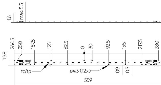
LLE 20x560mm 2400lm LV SNC4
