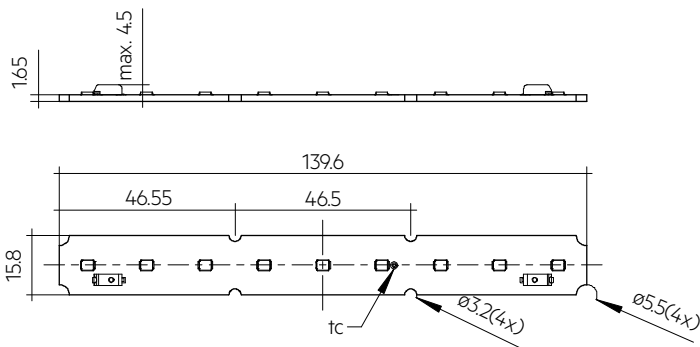
LLE 16x140mm 650lm HV ADV6
