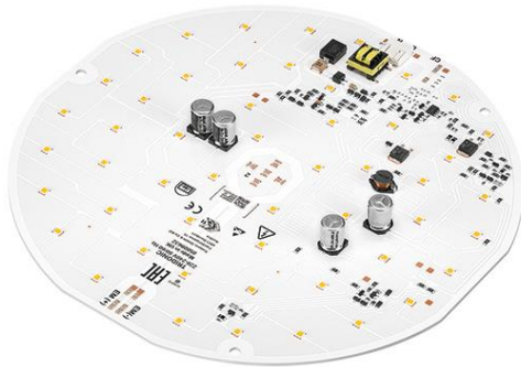
CLE AC G2 220mm 2500lm ADV
