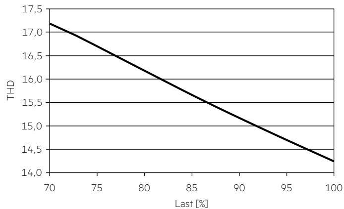
4.3.5 THD in Abhängigkeit von der Last
