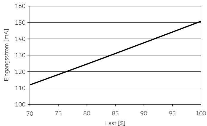
4.3.4 Eingangsstrom in Abhängigkeit von der Last
