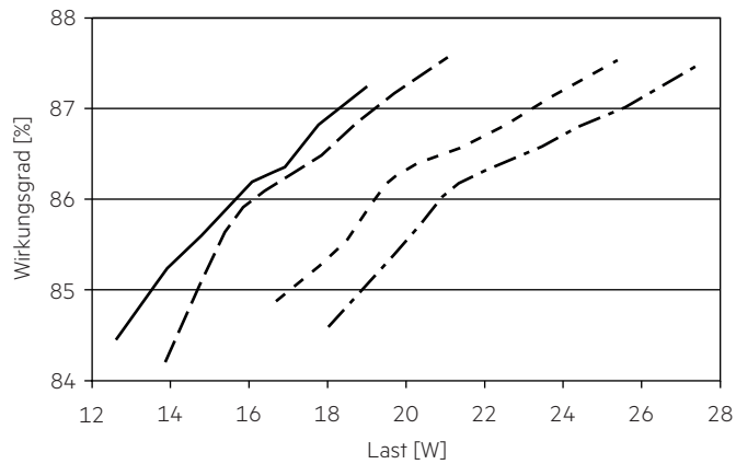
4.1.1 Wirkungsgrad in Abhängigkeit von der Last
